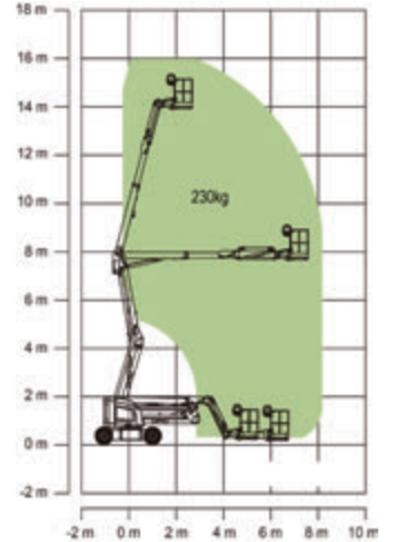
ZA14NJE/ZA14NJE-Li Hareket Aralığı
