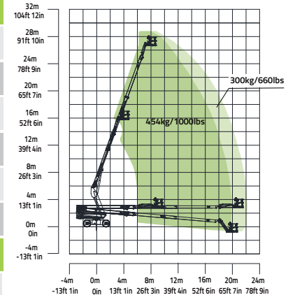
ZT26JE Hareket Aralığı
