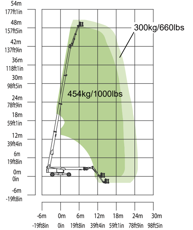
ZT51JEH-V Hareket Aralığı
