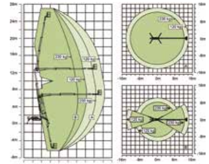
Hareket Aralığı ZX27AE
