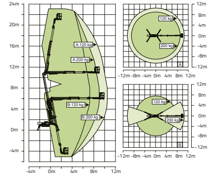
Hareket Aralığı ZX23AE
