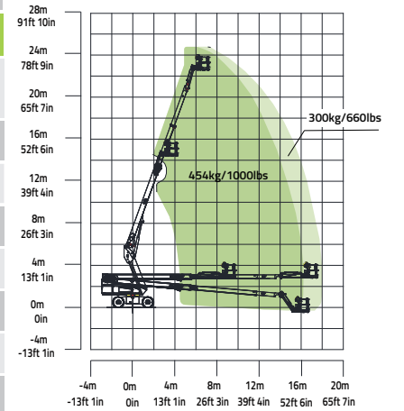
ZT22JE Hareket Aralığı
