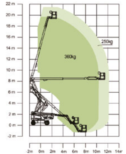
Hareket Aralığı ZA20JERT/ZA20JERT-Li
