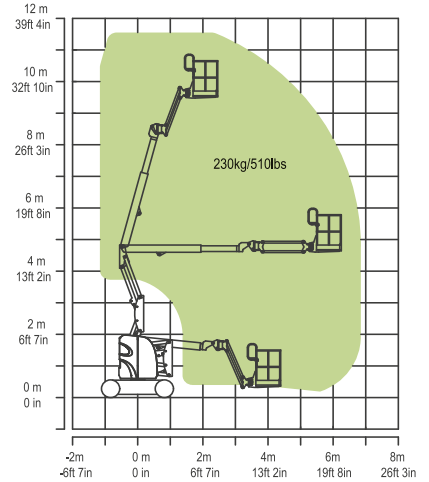
ZA10RJE Çalışma Diyagramı
