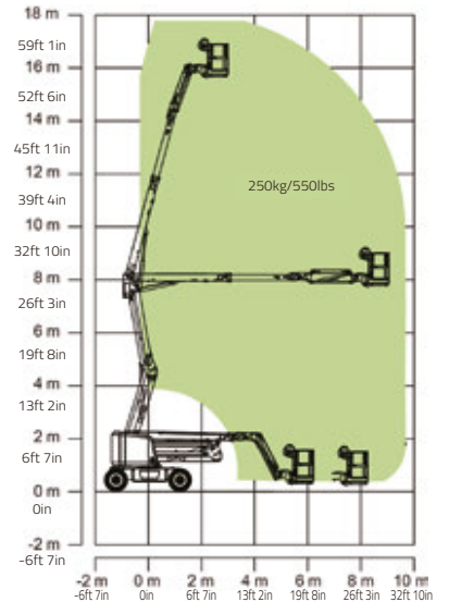
Hareket Aralığı ZA16JERT/ZA16JERT-Li
